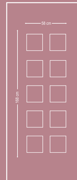
ET820012 Σχέδιο δέκα τζάμια δέλτα ματ καιί λευκό χιαστί Ten windows delta mat decorative lattice white x-shaped design
