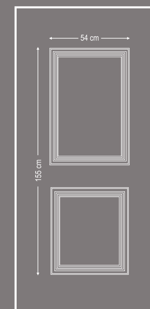
ET820724 Σχέδιο χωρίς τζάμι – διπλής όψης No glass – two sided design
