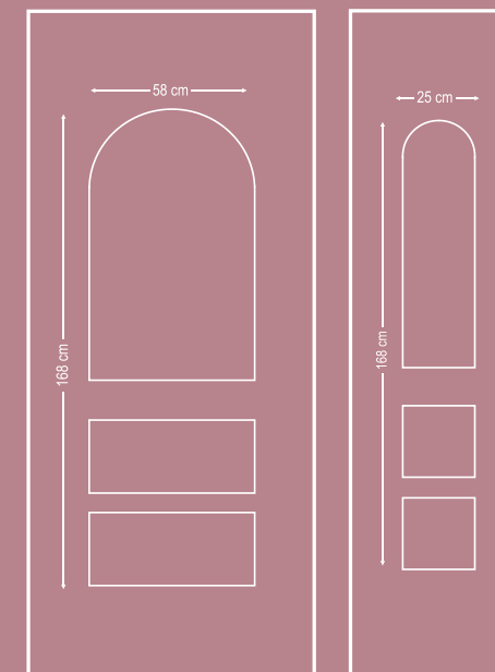
ET820030 Σχέδιο ένα τζάμι δέλτα ματ καιί λευκό ρόμβο One window delta mat decorative lattice white rhombus design
