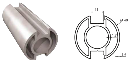
Κολώνα 2 καναλιών (40x1,6 mm) Ø40 Strut with 2 canals (40x1,6 mm) Ø40
