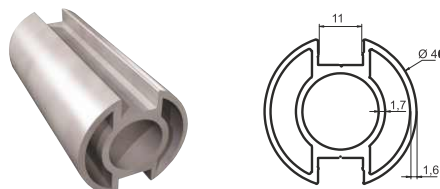
Κολώνα 2 καναλιών (40x1,6 mm) Ø40 Strut with 2 channels (40x1,6 mm) Ø40
