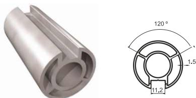
Κολώνα με 1 κανάλι Ø40 Strut with 1 channel (40x1,5 mm) Ø40
