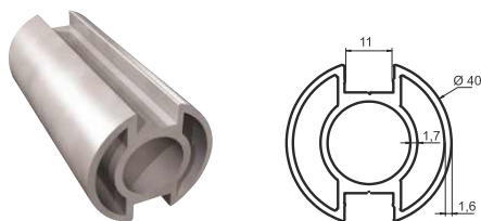
Κολώνα 2 καναλιών (40x1,6 mm) Ø40 Strut with 2 channels (40x1,6 mm) Ø40
