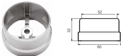
Επιτοίχια φλάντζα κουραστής Ø50 Wall flange Ø50
