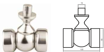
Ρυθμιζόμενος γωνιακός σύνδεσμος κουραστής Ø50 Adjustable support for upper profile (for corner strut) Ø50
